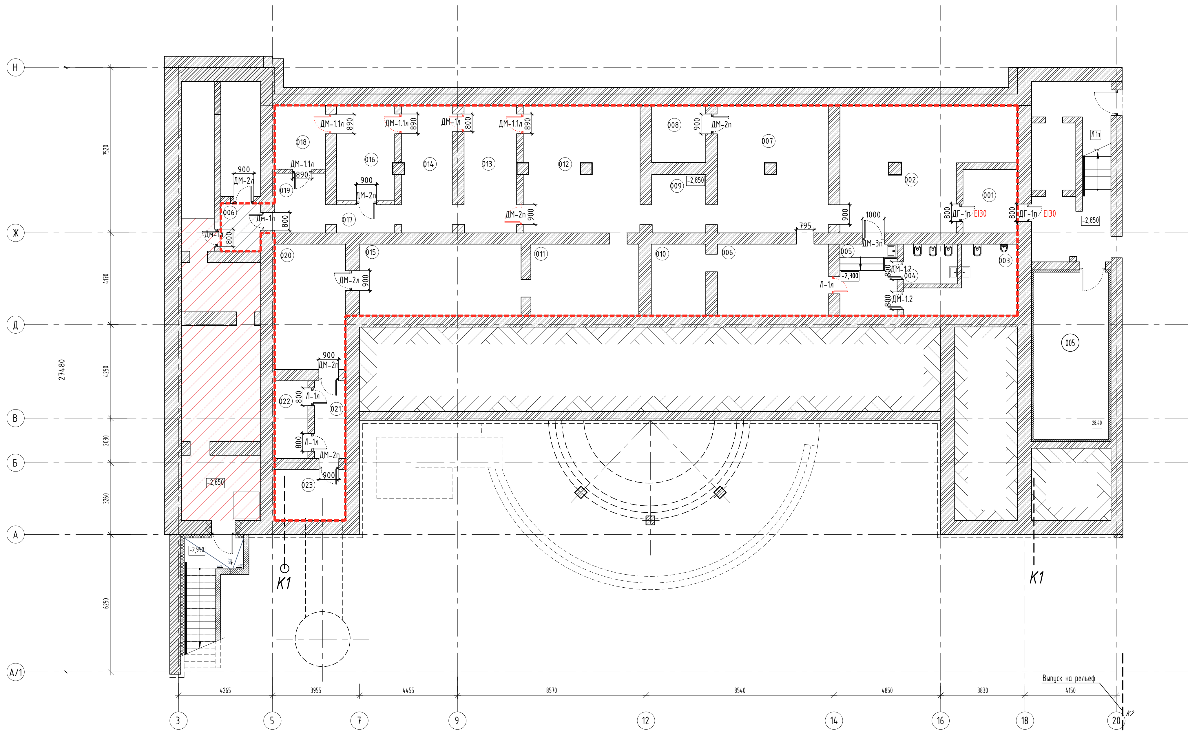
Фрагмент плана подвала на отм. -2,850. Укрытие. Маркировочный план
