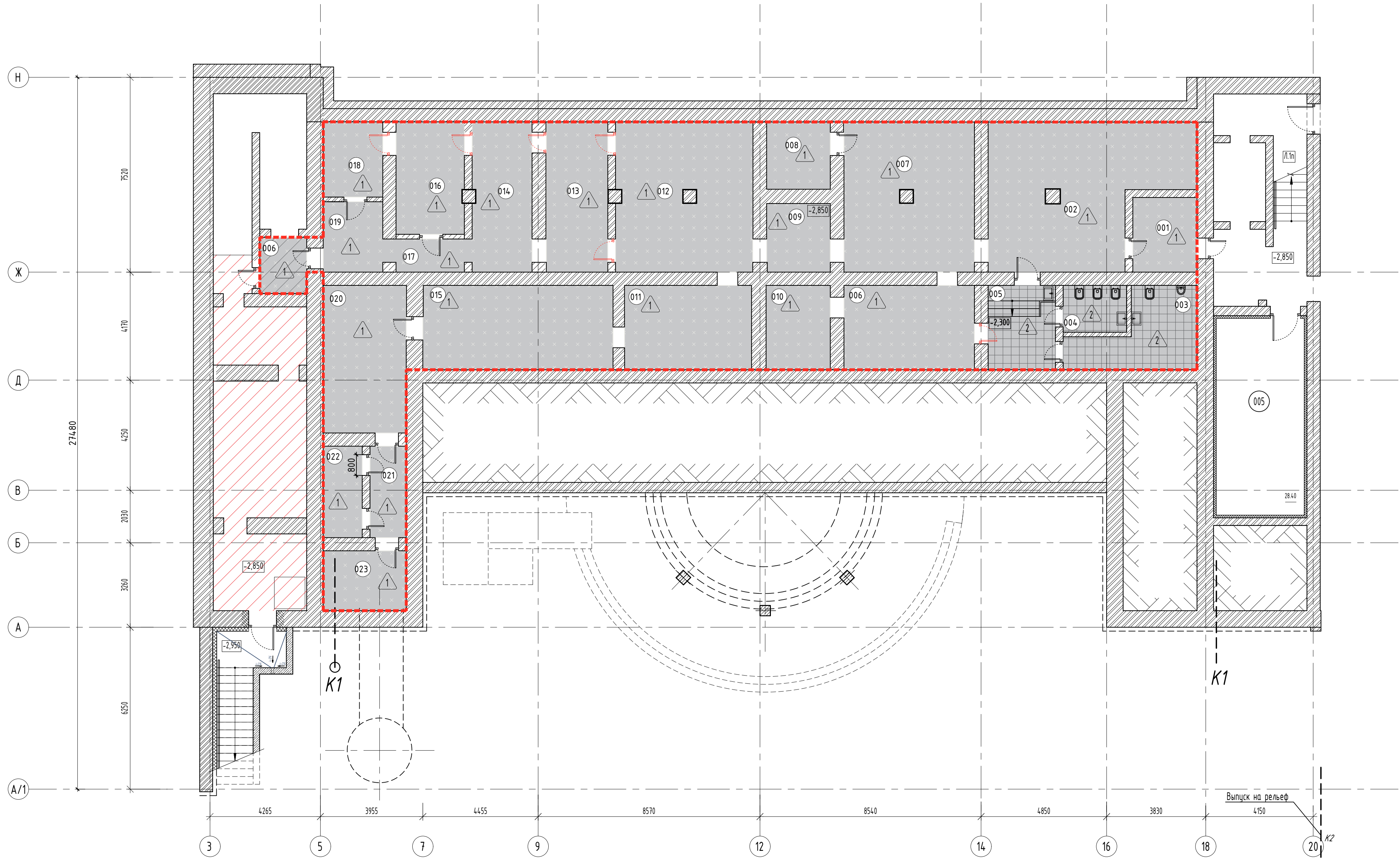
Фрагмент плана подвала на отм. -2,850. Укрытие. Отделка пола
